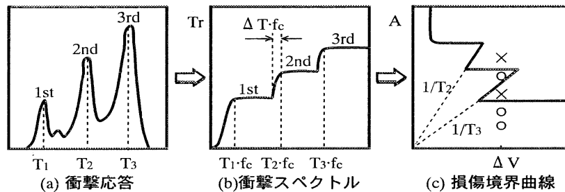
図3 衝撃応答における複数のピークと損傷境界曲線の関係
