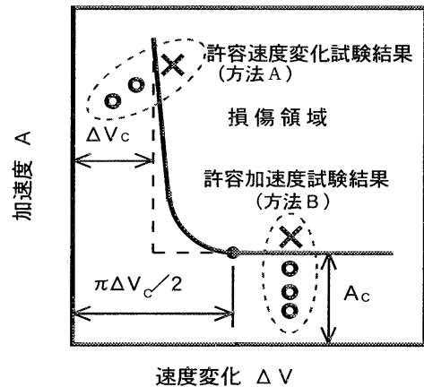
図2 損傷境界曲線と衝撃強さ試験方法
