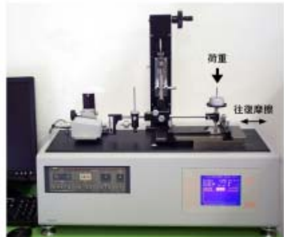
図1 往復動摩擦摩耗(表面性)試験機
