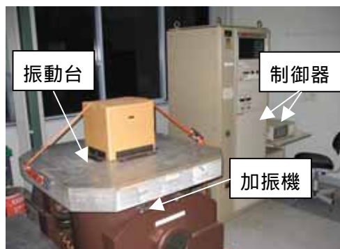
図1 振動試験機
