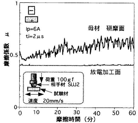
図5 摩擦試験における摩擦係数の時間変化
