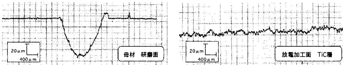
図6 摩擦試験後の摩耗痕の形状
