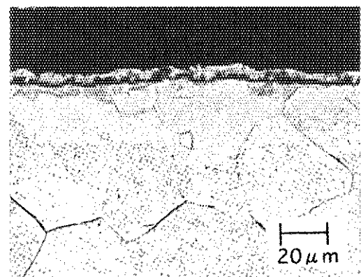
図3 加工面の断面組織
