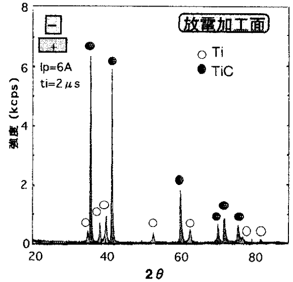
図4 加工表面からのX線回折図形
