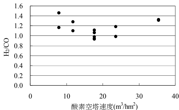
図6 H 2 /CO と酸素空塔速度の関係
