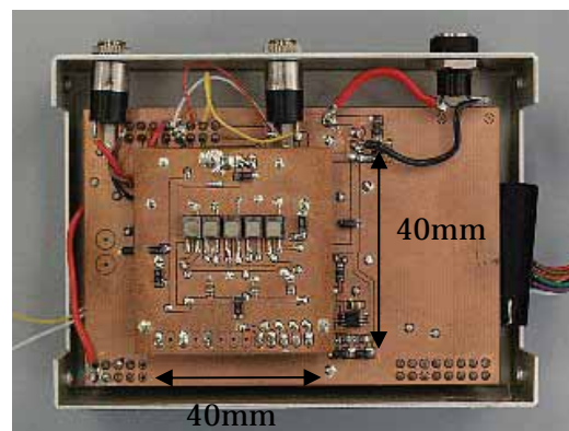
図5 二次元位置計測システム
