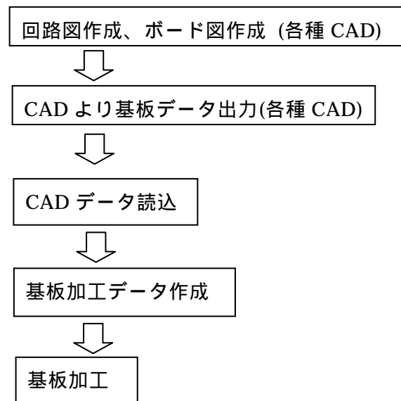
図2 基板作成の流れ
