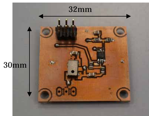
図4 回路部品実装後の基板
