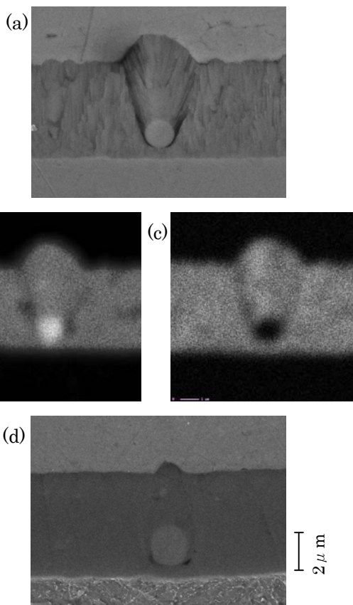
図3 CrN 皮膜断面の SEM 写真
