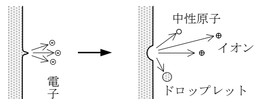
図 1 ドロップレット発生の概略図
