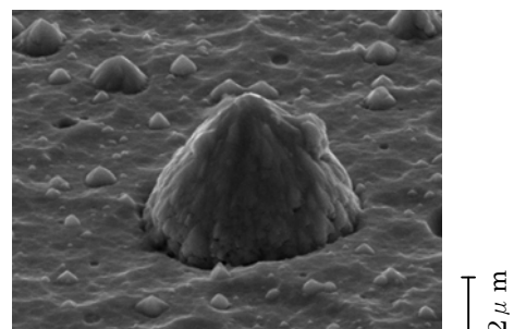
図 2 CrN 皮膜表面の SEM 像 ( V_b = -50V )
