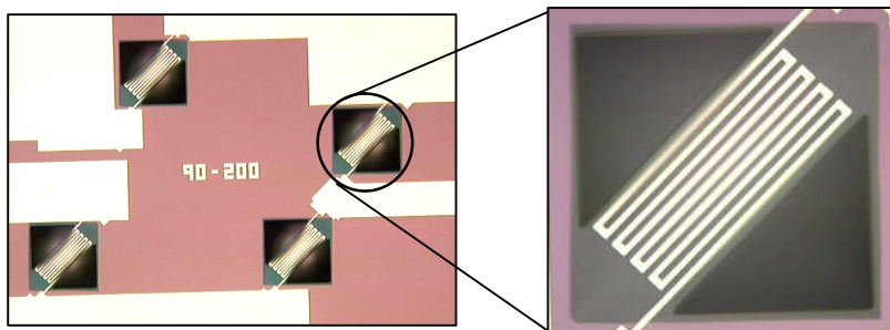
試作予定の抵抗ボロメータ型赤外線センサ
