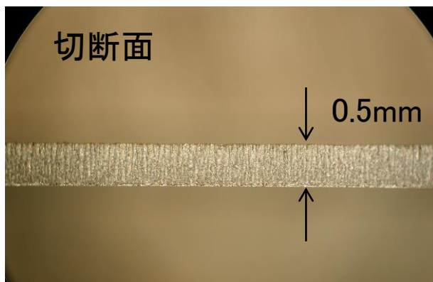
シリコンウエハ 厚さ0.5mm レーザパワー20W, 切断速度10mm/s
